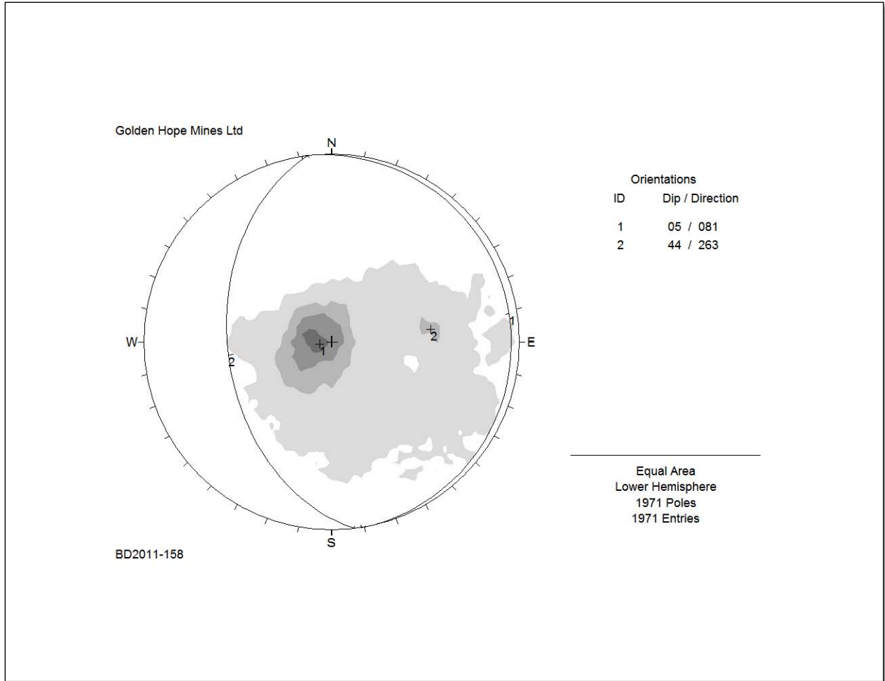
Figure 2. BD2011-158 -- Stereonet showing one set of flat lying structures plus a smaller set of moderately dipping structures. Stereonet montrant une famille de structures sub-horizontales plus une famille de pendage moyen.
